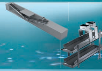
Kastenverarbeitung / crate handling Unterflurförderer und Doppelstockhöhenförderer Underfloor conveyor and Double-decker conveyor
