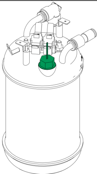
Bisheriger Boiler mit Temperaturfühler mit integrierter Verschraubung
