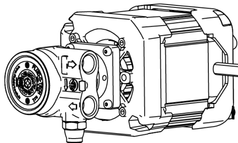
Alternative Flügelzellenpumpe:
