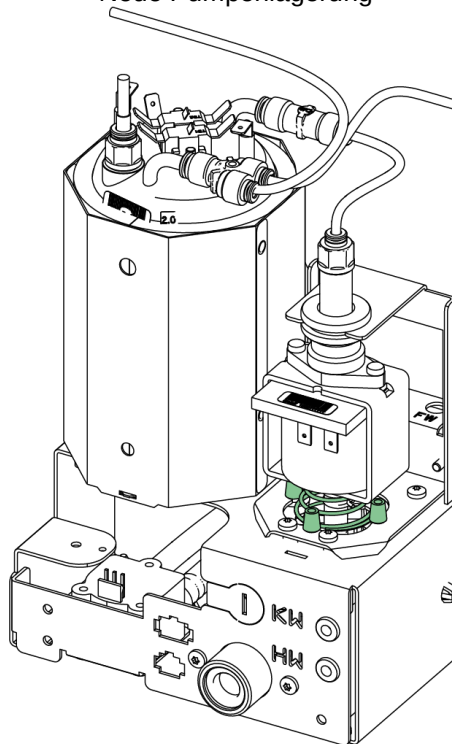
Neue Druckfeder
