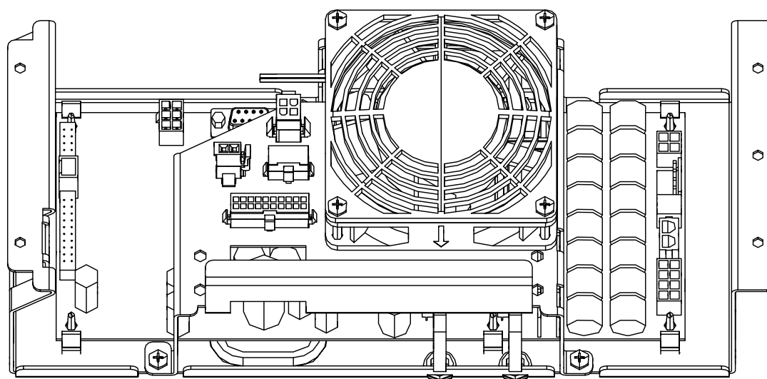
701 04 307 00 Steuerungsträger kpl mont IMAX 2 Microschritt
