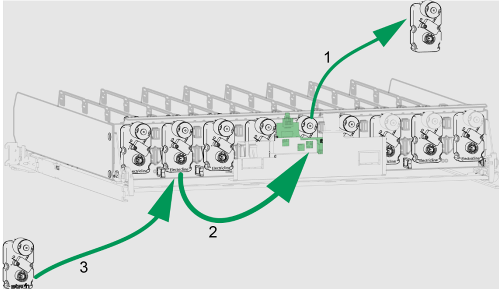
Abbildung 1 Warenfach mit ElectricLine Motoren – Bitron Motor als neues Ersatzteil
