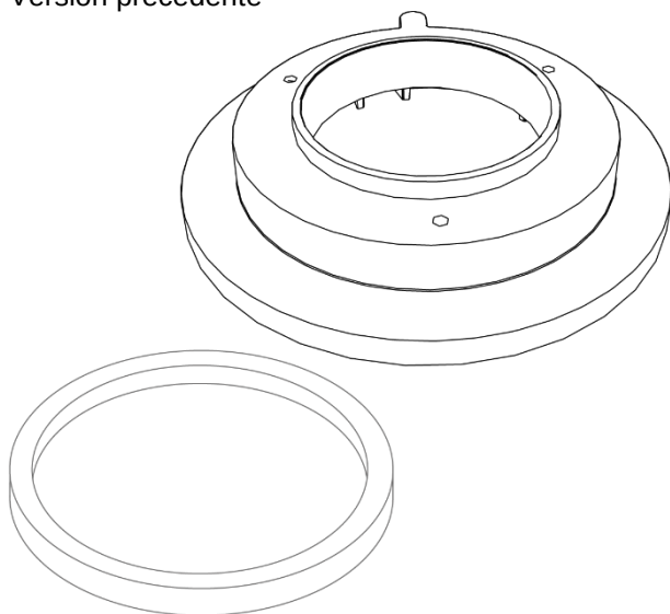
Bague de réglage de la mouture (joint torique nécessaire)
