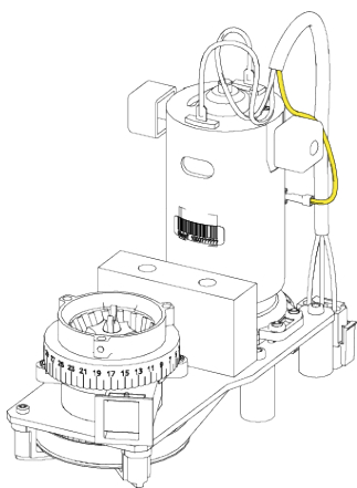
Ancien moulin encastrable
