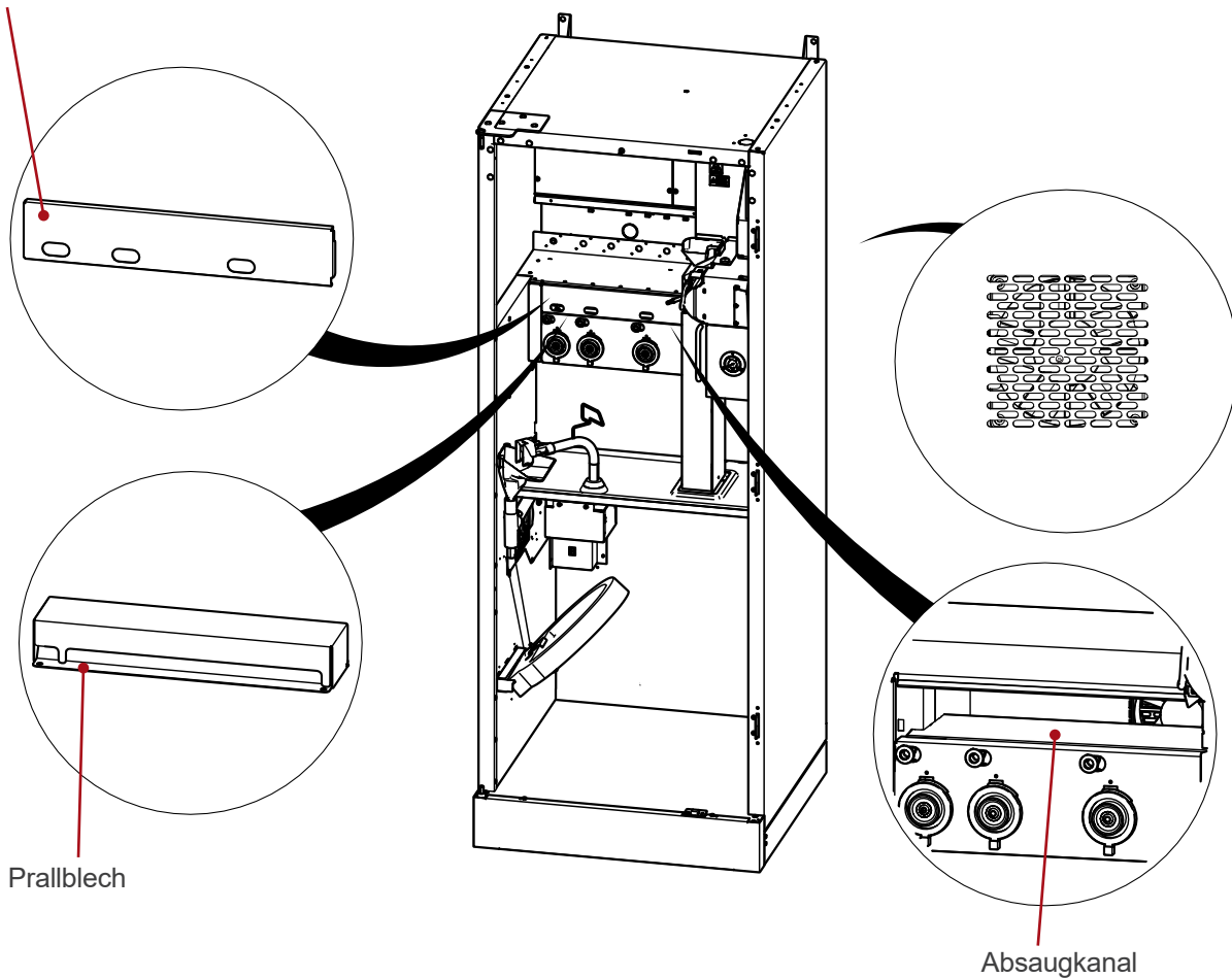
Querträger-Absaugung
