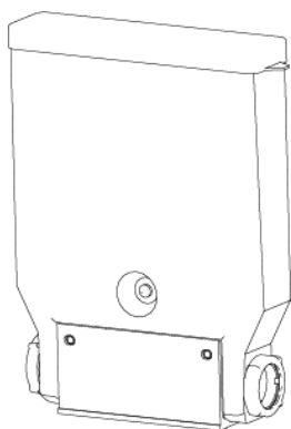
Bisherige Behälterausführung
